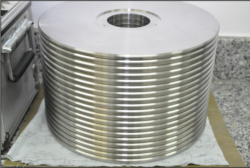
Zestaw obciążników do stanowiska wzorcowego o zakresie pomiarowym do 100 MPa.
